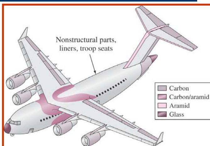
Empleo de materiales polímeros/compuestos en la aviación
